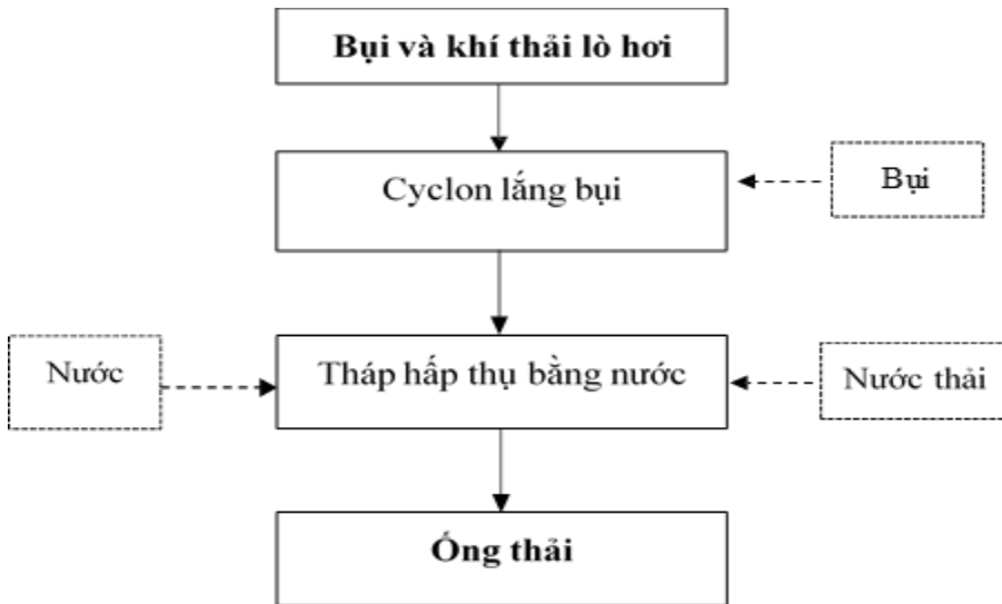
Hình 2.1. Sơ đồ quy trình công nghệ xử lý bụi và khí thải lò hơi
